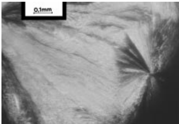
Slika 3: Pahlja-asta slika C3-diola, ki nastane pri ohlajanju izotropne faze v teko-ekristalno, T = 114^{\circ}\text{C} , pove-ava 125-kratna
